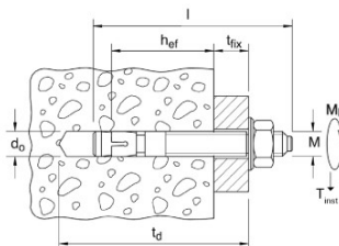
Anclaje FWA
